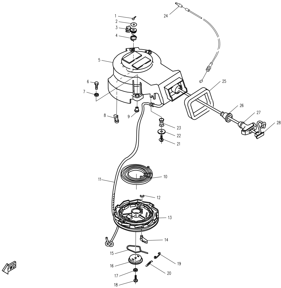
图7 起动机
