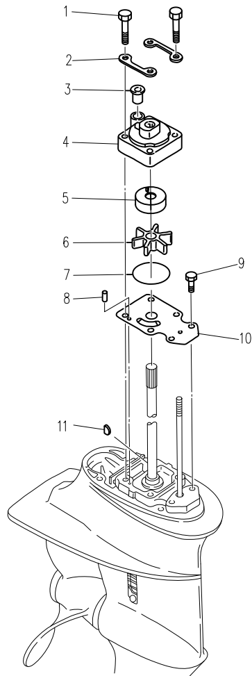
图19 水泵
