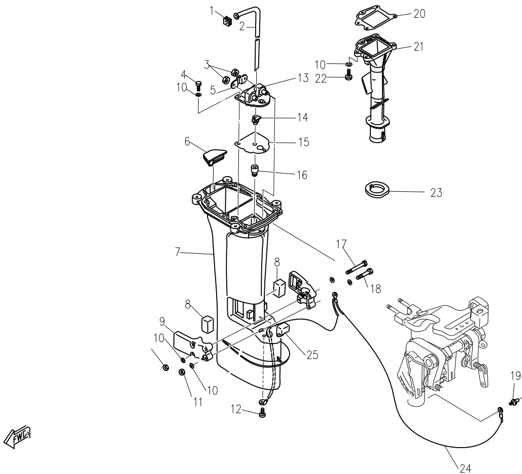
FIG. 15 UPPER CASE AND EXHAUST MANIFOLD 图15 水上排气
