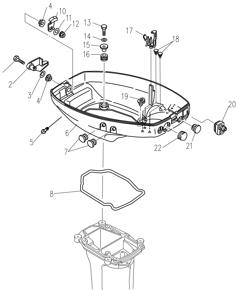
FIG. 10 BOTTOM COWLING 图10 底罩
