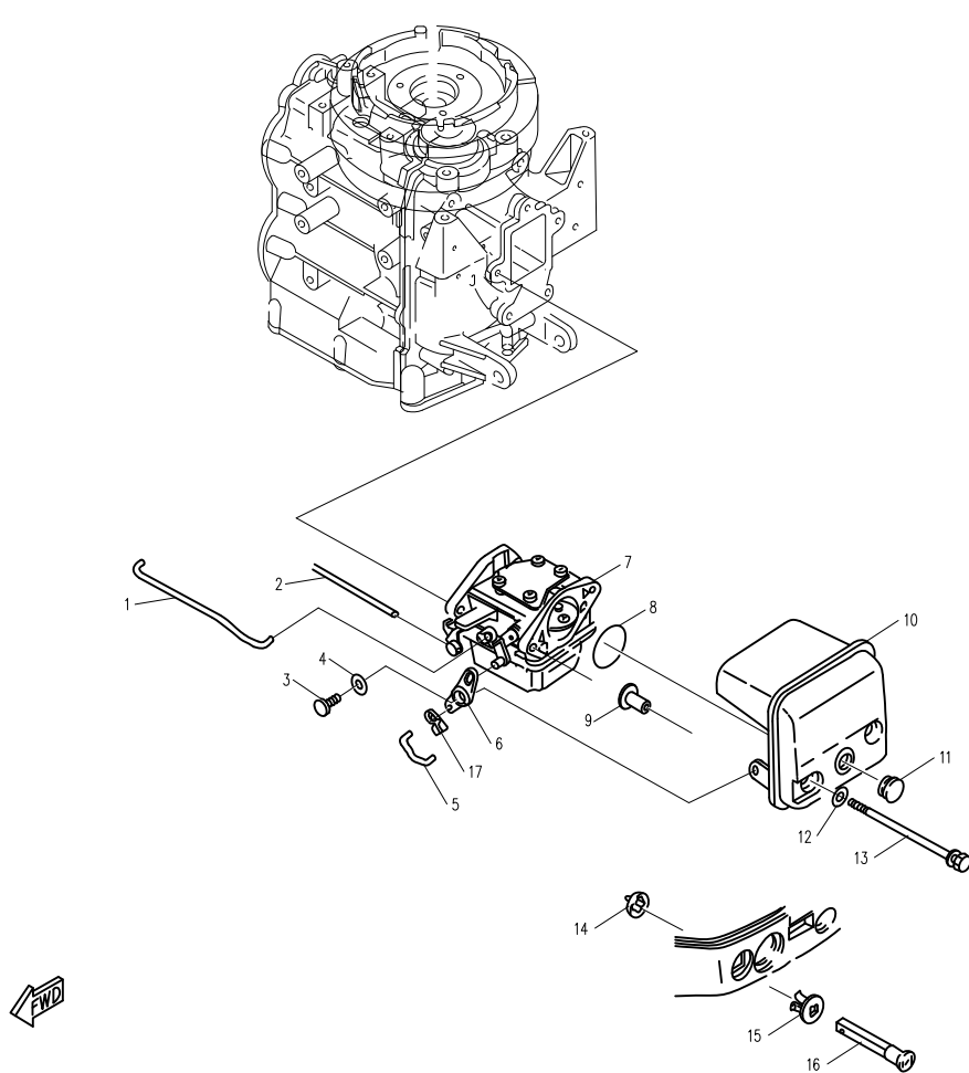
FIG. 6 INTAKE 图6 进气系统
